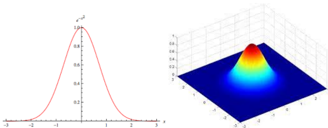
Figure 1: Gaussův integrál I (vlevo) a jeho 2D varianta I^2 (vpravo).
