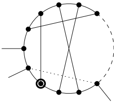
(d) v has type II.
