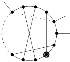
(d) Type II.
