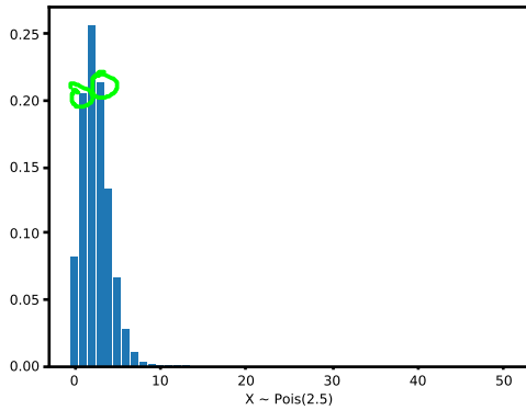
(a) Poissonovo rozdělení s parametrem \lambda .
